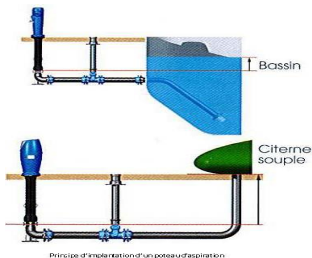
Principe d'implantation d'un poteau d'aspiration
