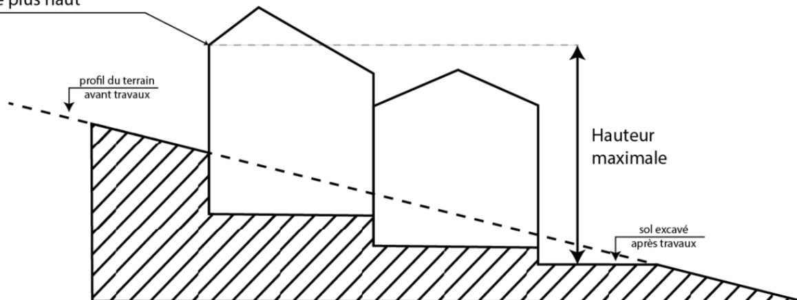
cas d'une construction composée de multiples corps bâtis en pente
