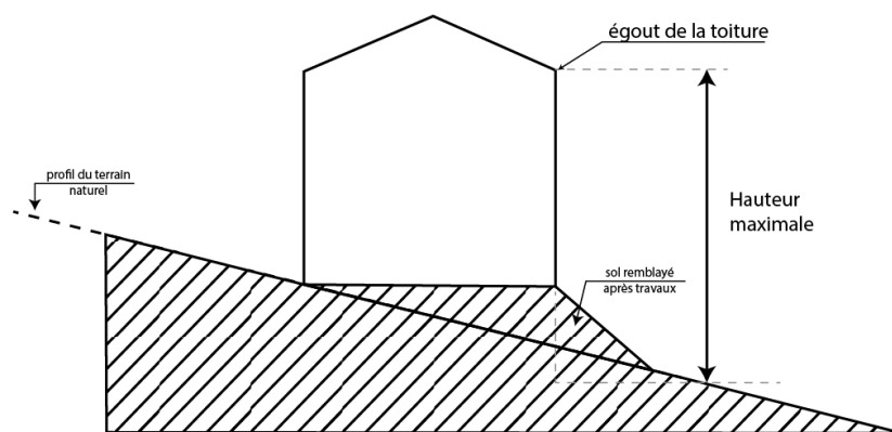
cas d'une construction avec sol remblayé
