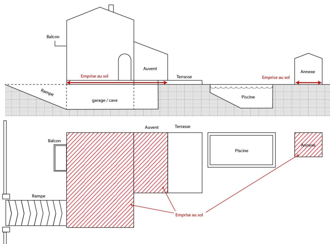
Schéma emprise au sol
