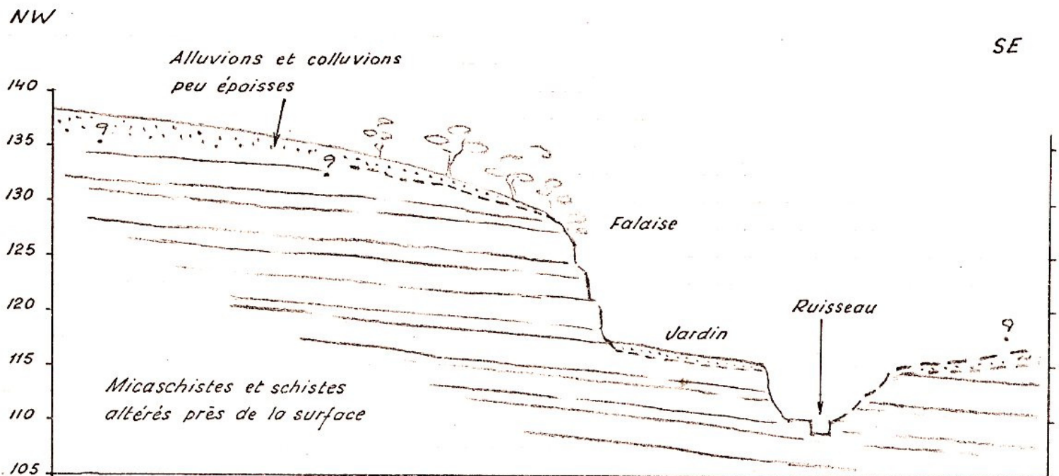
COUPE 2
