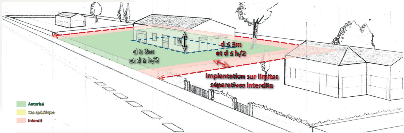
Schéma 13 : Hauteur des constructions, cas particulier (Article UX10, Paragraphe 3) :
