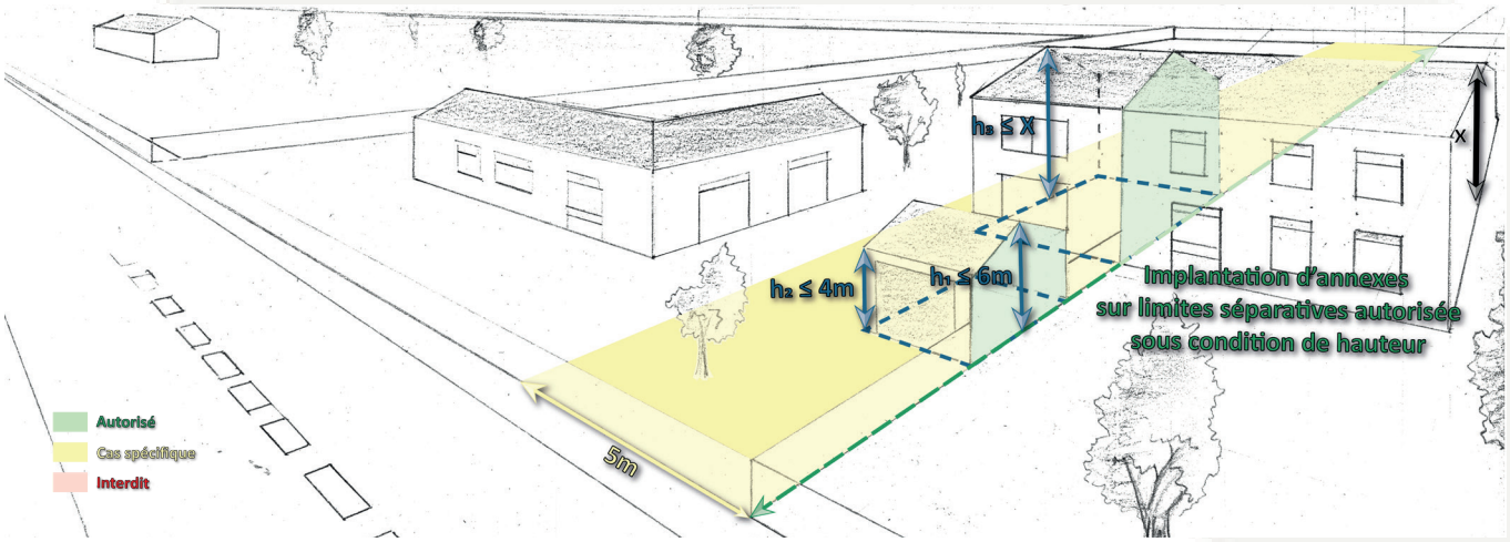
Schéma 25 : Hauteur des constructions, cas particulier (Article N10, Paragraphe 3) :
