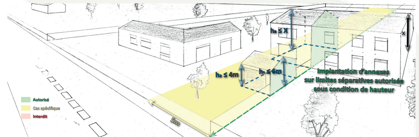
Schéma 17 : Hauteur des constructions, cas particulier (Article AU10, Paragraphe 3) :
