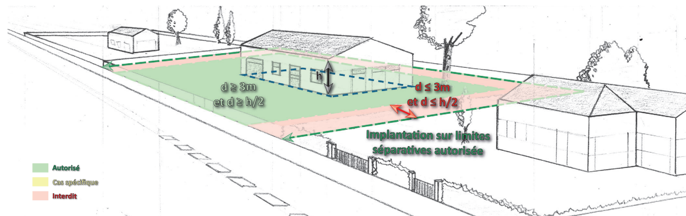
Schéma 15 : Implantation des constructions par rapport aux limites séparatives (Article AU7)
