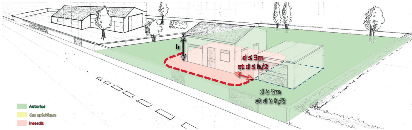
Schéma 12 : Implantation des constructions les unes par rapport aux autres sur une même propriété (Article UX8, Paragraphe 1) :
