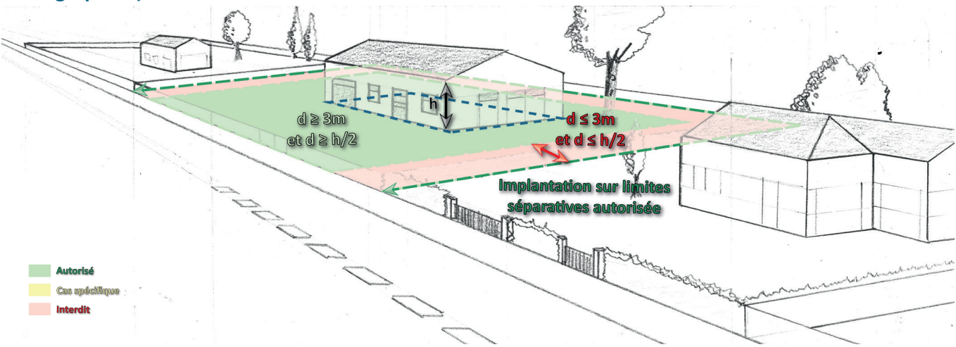
Schéma 19 : Implantation des constructions par rapport aux limites séparatives (Article A7, Paragraphe 1)
