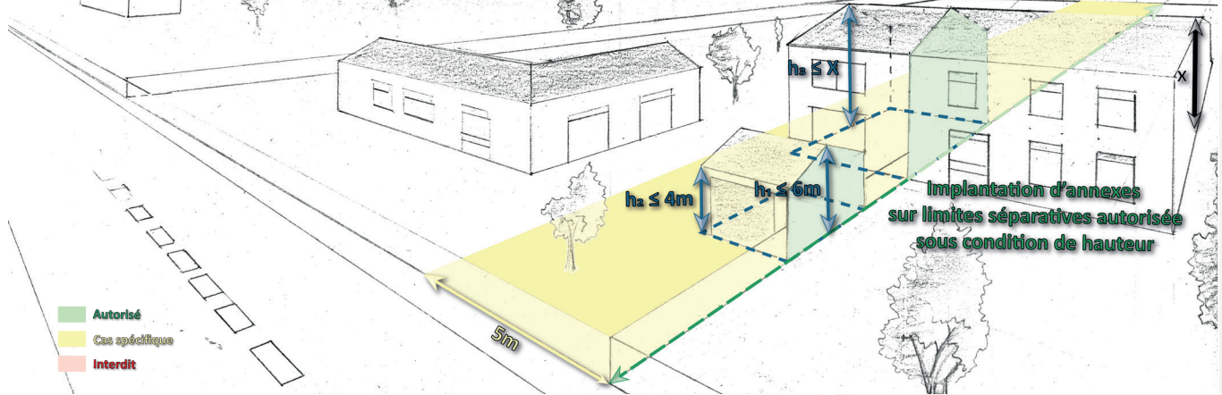
Schéma 13 : Hauteur des constructions, cas particulier (Article UX10, Paragraphe 3) :
