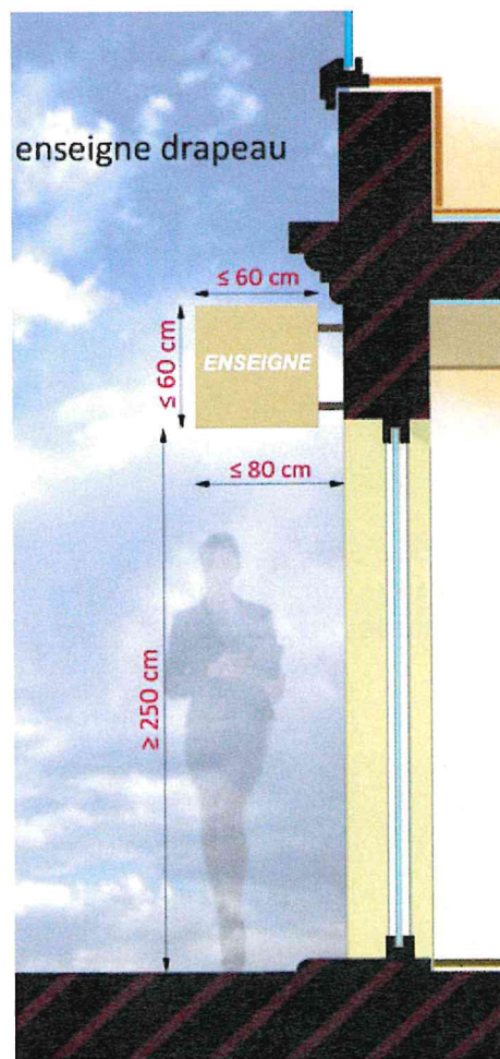
Principe d'implantation de l'enseigne drapeau
