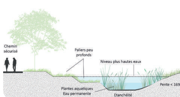
Exemple de bassin avec retenue d'eau
