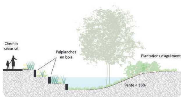
Exemple de bassin avec infiltration
