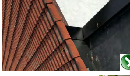
Bonne pratique : Détail de remontée d'étanchéité sous toiture existante
