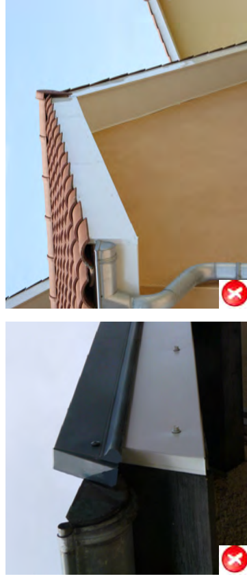
Exemple d'isolation par l'extérieur (Sarking) (ill. extrait de l'exposition «La rénovation thermique» EIE Bretagne)
