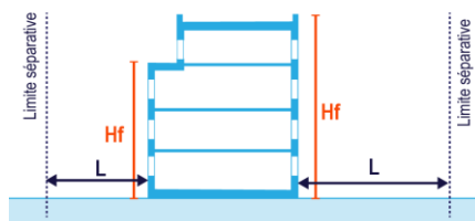
Façades avec baie : L \geq Hf et L \geq 8m
