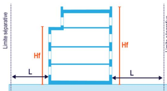
Façades avec baie : L \geq H_f - 3m et L \geq 5m
