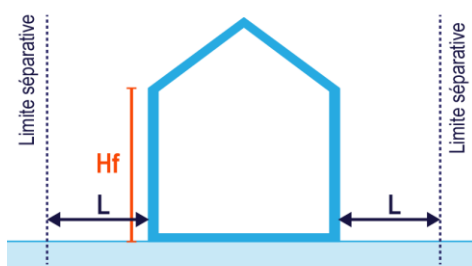
Façades sans baie : L \geq H_f/2 et L \geq 3m
