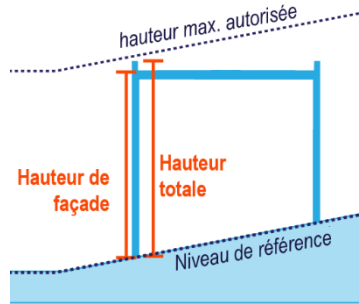
Cas des toitures terrasses sans attique
