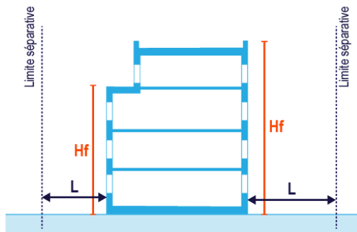
Façades avec baies : L \geq H_f/2 et L \geq 4m
