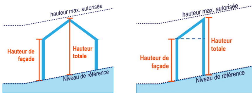
Cas des toitures à pente
