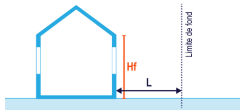
Façades avec ou sans baie : L \geq H_f et L \geq 8m
