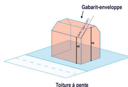
Toiture à pente
