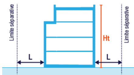
Façades sans baie : L \geq (Ht/2)-3m et L \geq 3m
