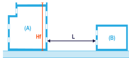
Façade avec baie : L \geq H_f(A) - 3m et L \geq 5m
