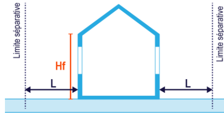
Façades avec baie : L \geq H_f et L \geq 8m
