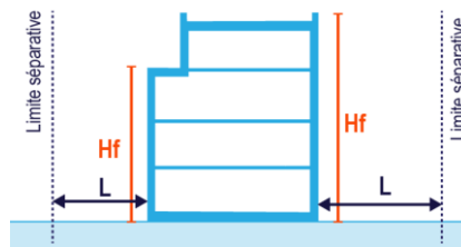
Façades sans baie : L \geq H_f/2 et L \geq 4m
