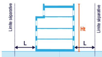
Façades avec baie : L \geq (Ht/2)-3m et L \geq 5m
