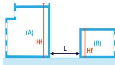
Façades sans baie : L \geq H_f/2(A) et L \geq 3,50m
