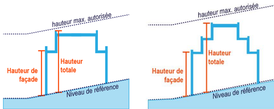
Cas des toitures terrasses avec attique
