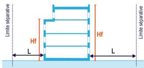
Façades avec baie : L \geq H_f et L \geq 6m
