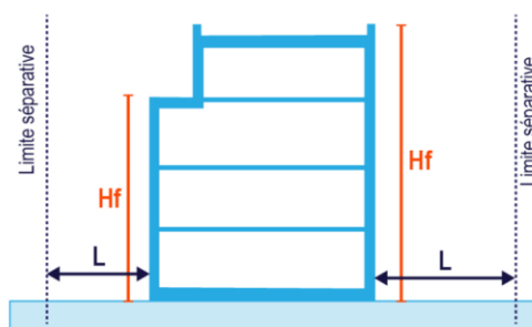
Façades sans baie : L \geq (H_f/2) - 3m et L \geq 5m
