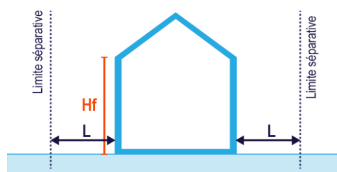
Façades sans baie : L \geq \frac{3}{4} H_f et L \geq 6m
