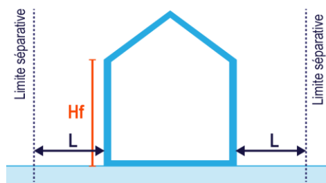
Façades sans baie : L \geq H_f/2 et L \geq 3m
