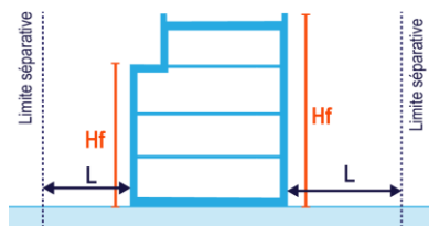
Façades sans baie : L \geq Hf/2 et L \geq 4m
