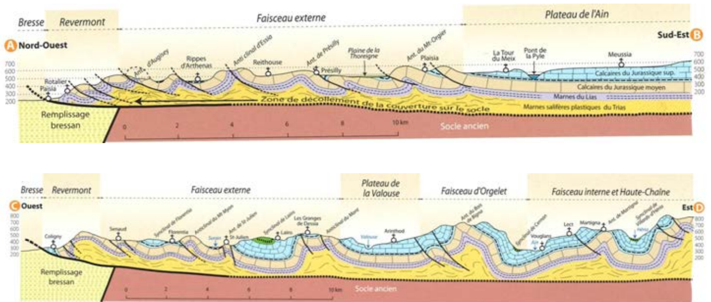
Coupes géologiques de la Petite Montagne du Jura
