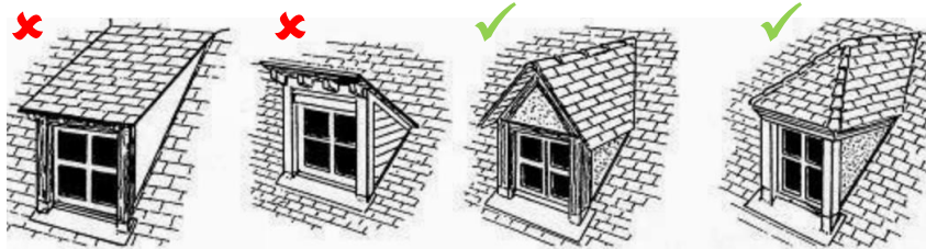
De gauche à droite : lucarne rampante, lucarne retroussée, lucarne à deux pans dite jacobine, lucarne à croupe dite capucine
