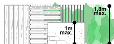
1,80m max. si transparence de la clôture
