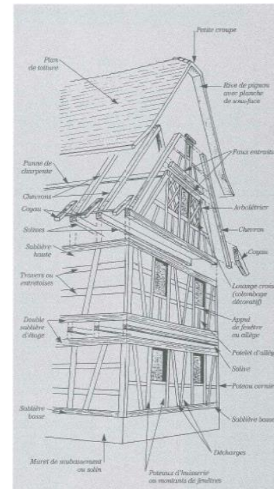
Éléments constructifs de la maison à pans de bois Source : Les maisons d'Alsace – T.Fischer et C. Fuchs
