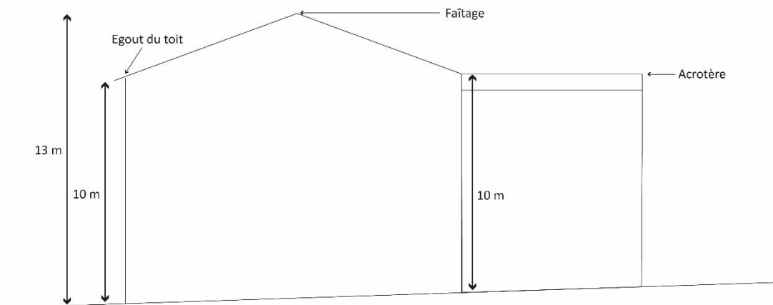
Figure 13 _ Hauteur maximale en tout point vis-à-vis du terrain d'origine
