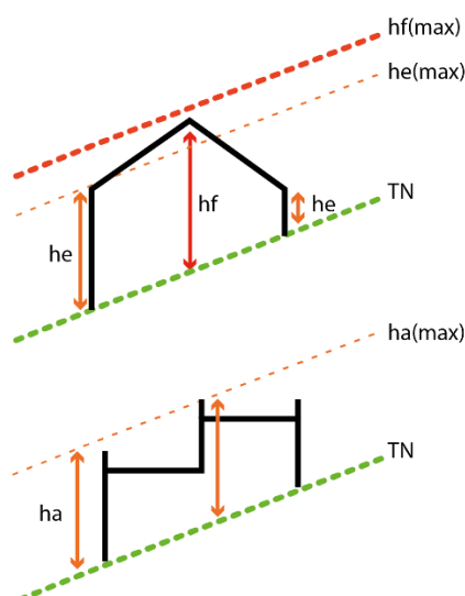
Figure 20 Principe de calcul de la hauteur (avec TN le terrain naturel avant travaux, he la hauteur à l'égout, hf la hauteur au faîtage, ha la hauteur à l'acrotère et h_{max} la hauteur référence du PLUiH)
