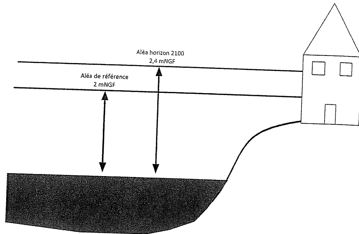
Représentation schématique des niveaux marins de référence
