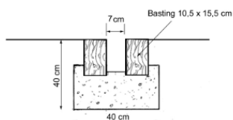
Caniveau bois pour traversées obliques
