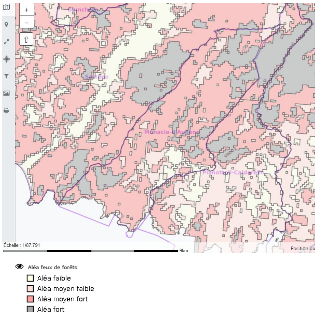
Figure 1 : Cartographie de l'aléa feu de forêt sur la commune de Monacia-d'Aullène (source : Les services de l'Etat en Corse-du-Sud)
