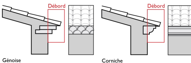
Schéma explicatif : Typologie de débords de toiture
