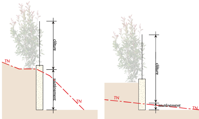
Schéma explicatif : Définition du soutènement
