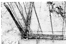
Noeud de chaînage - Continuité mécanique
