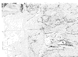
Extrait de carte géologique
