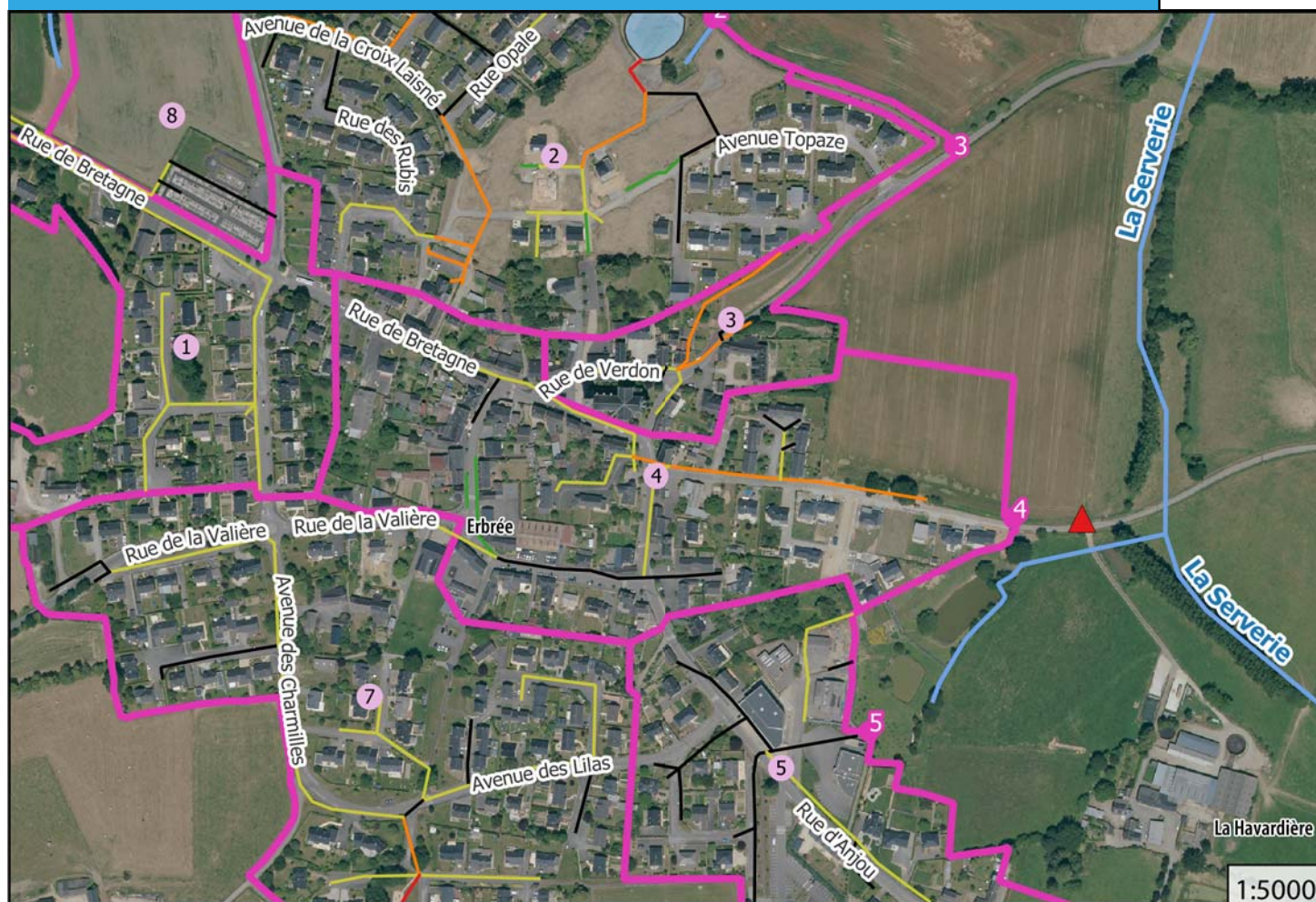
Carte du bassin versant n°4
