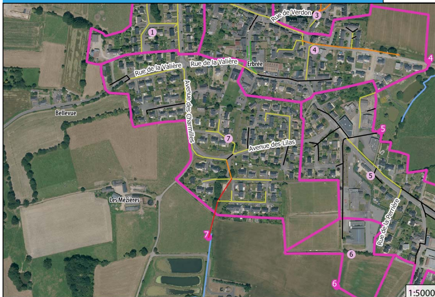
Carte du bassin versant n°7
