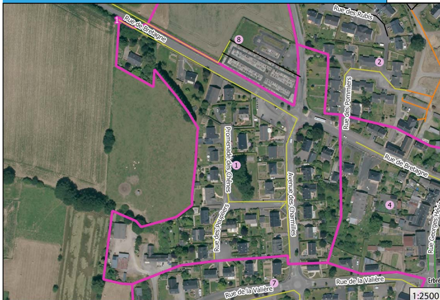
Carte du bassin versant n°1
