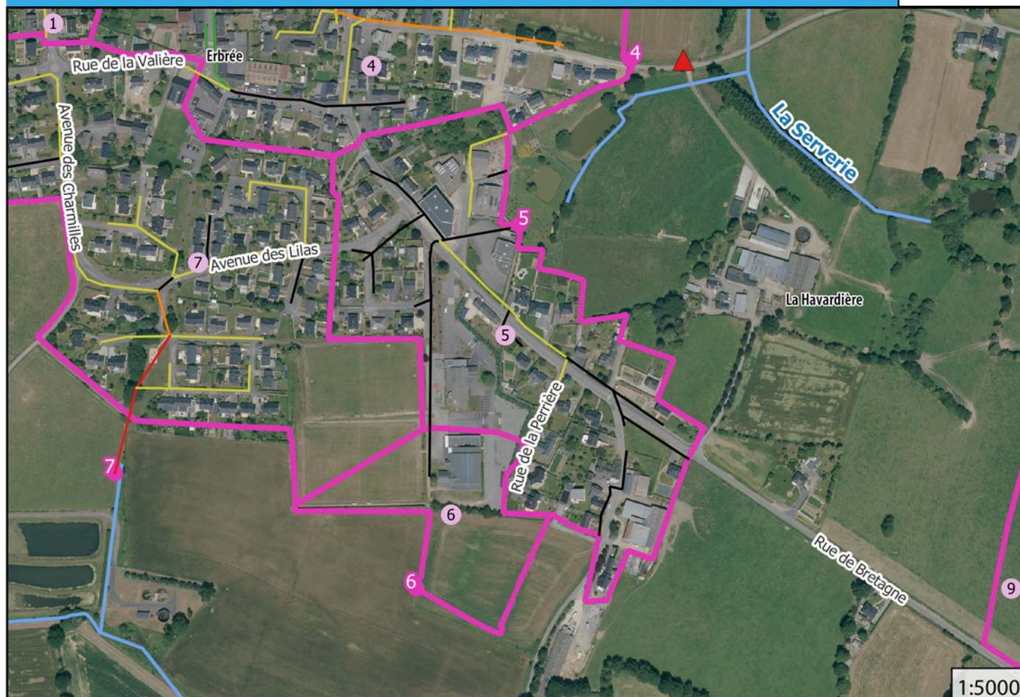
Carte du bassin versant n°5
