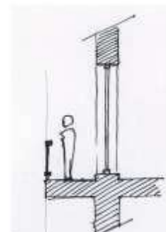
Garde-corps sur un seul plan
