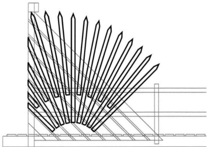
protection latérale en demi-rondins
