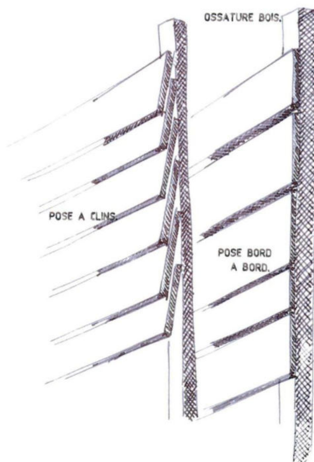
bardage de la cabane
