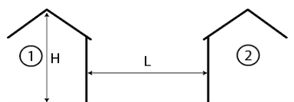
Cas où les murs 1 et 2 comportent des baies de pièces habitables
