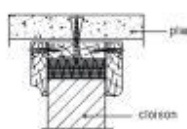
Liaison cloison-plancher (extrait des règles PS-MI)
