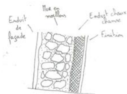
Coupe d'une isolation intérieure avec enduit chaux-chanvre
