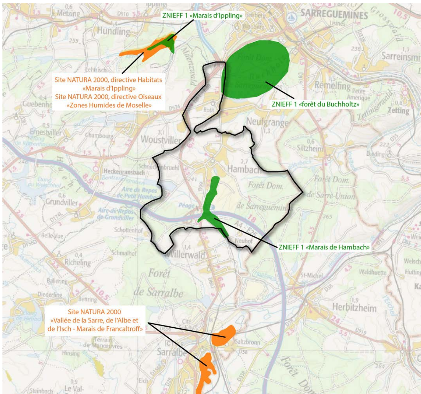
Localisation des espaces naturels protégés (ZNIEFF et NATURA 2000), sur le ban communal ou à proximité
