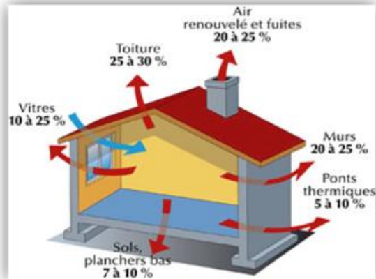
Les principales pertes d'énergie
