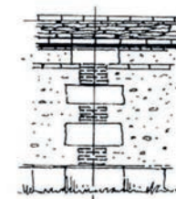
• MUR COMPOSITE CHAÎNE HARPÉE EN PIERRE DE TAILLE ET BRIQUE
