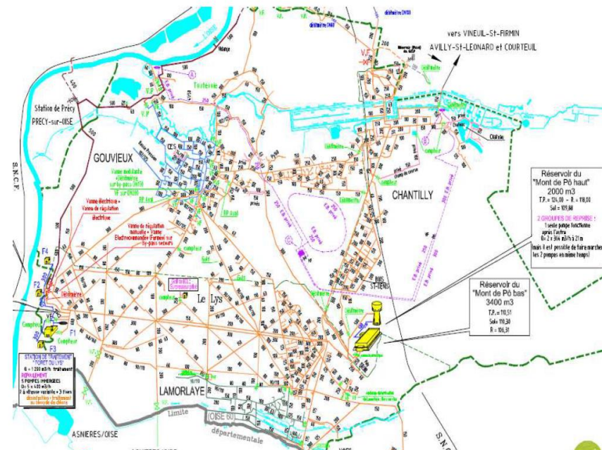
Schéma d'alimentation en eau potable – Source : Rapport déléguataire Eau 2018
