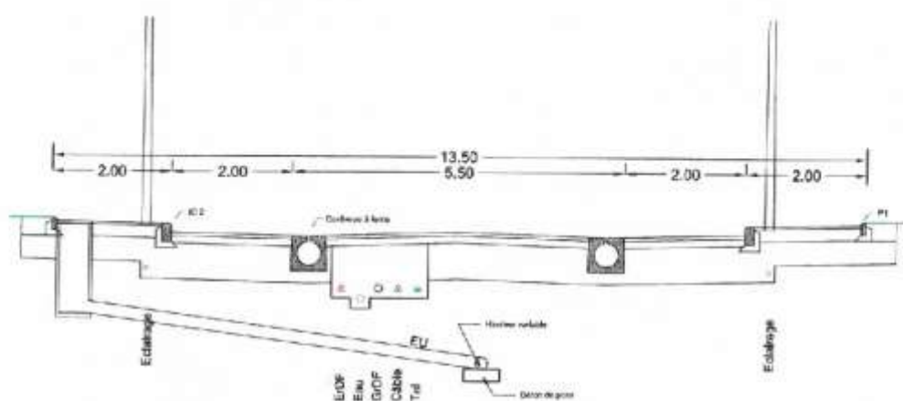
COUPE - VOIRIE PRINCIPALE
