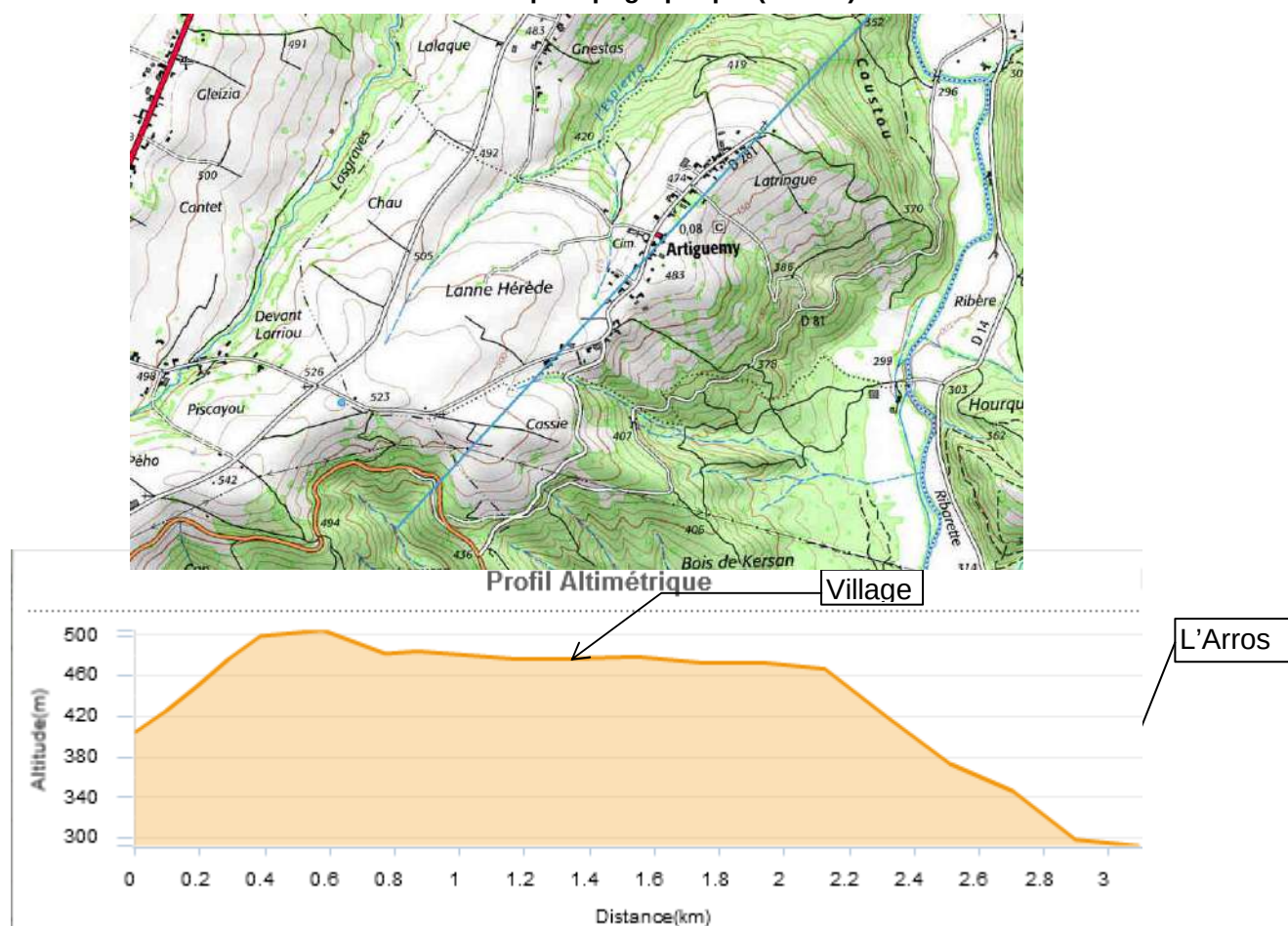
Illustration 1: Coupe topographique (SO-NE)
