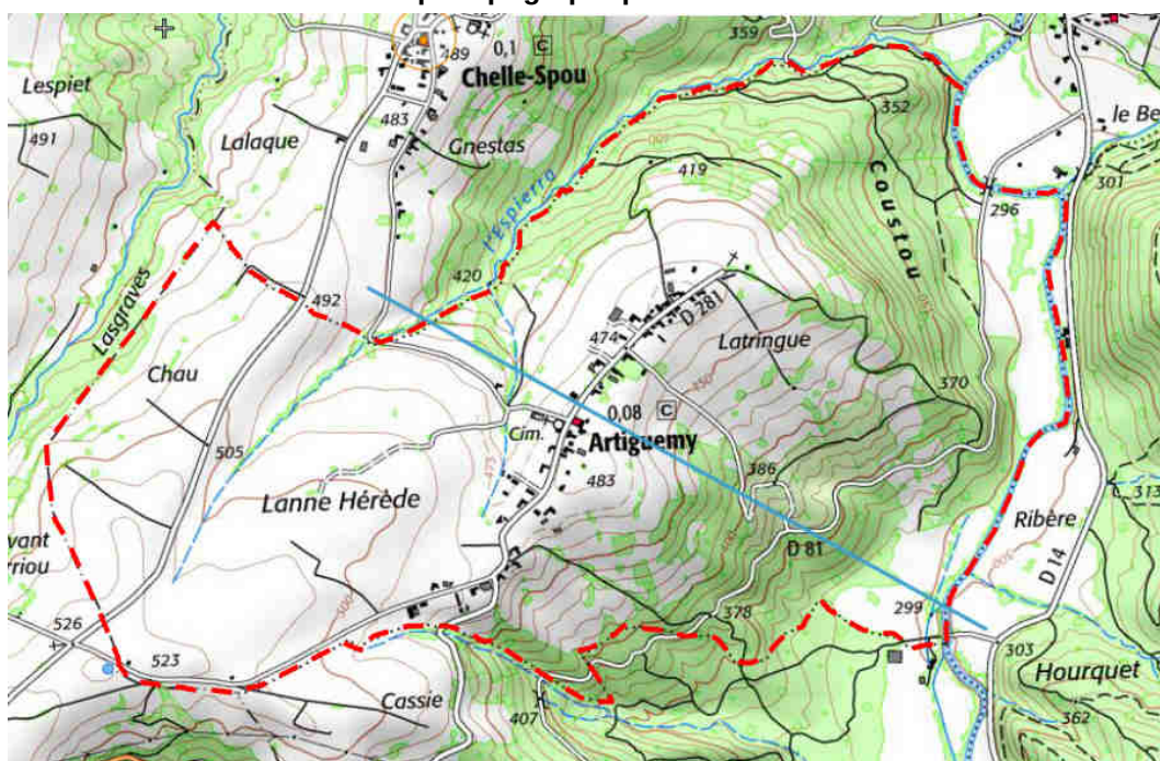
Illustration 2: Coupe topographique Nord-Ouest/Sud-Est
