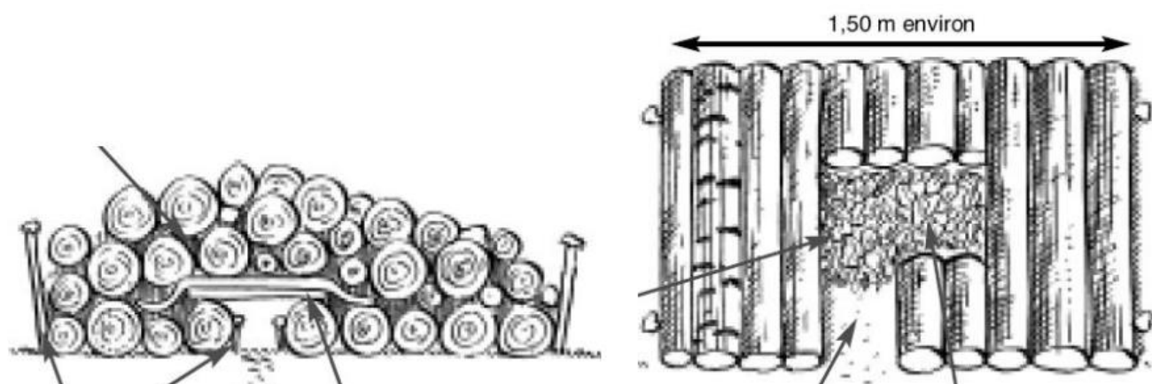
Figure 52 : Schéma de gîte artificiel « tas de bois » pour la petite faune terrestre
