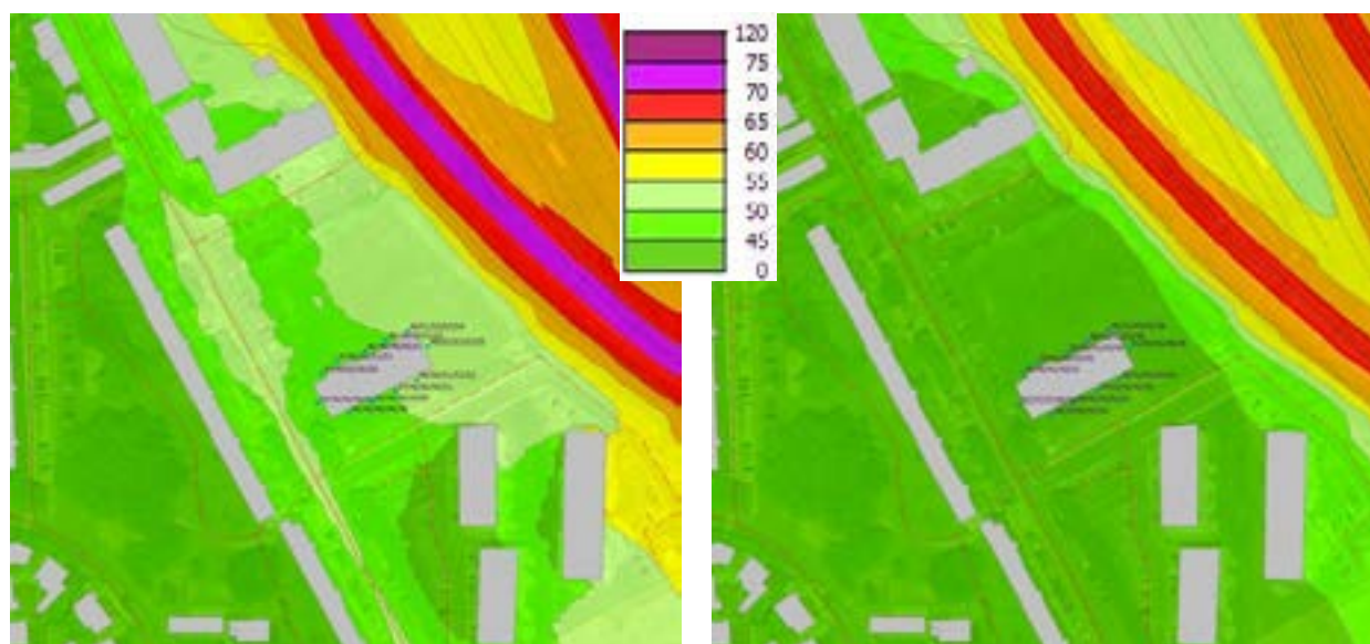
Situation de projet - Carte de niveaux sonores diurnes LAeq(6h-22h) estimés à 4m du sol, en dB(A) Valeurs en façades et par étage RdC / R+1 /.../ R+4.
