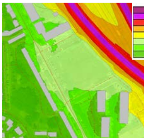
Etat initial - Carte de niveaux sonores diurnes LAeq(6h-22h) estimés à 4m du sol, en dB(A)
