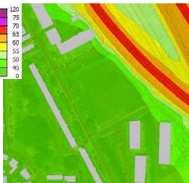
Etat initial - Carte de niveaux sonores nocturnes LAeq(22h-6h) estimés à 4m du sol, en dB(A) Seuil OMS en vert foncé (<44/ 45 dB(A))
