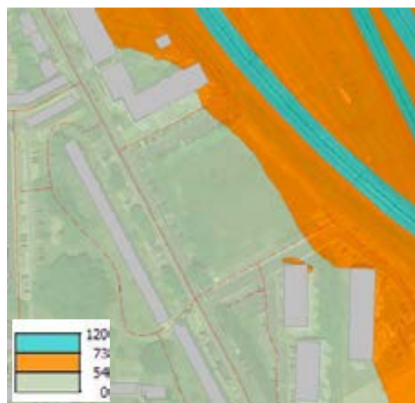
Etat initial - Carte de seuils Lden OMS et zones de PNB estimés à 4m du sol, en dB(A)
