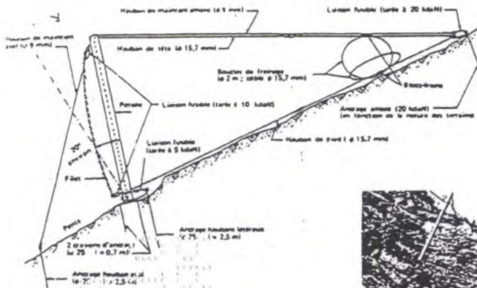
Ecrans de filets métalliques
