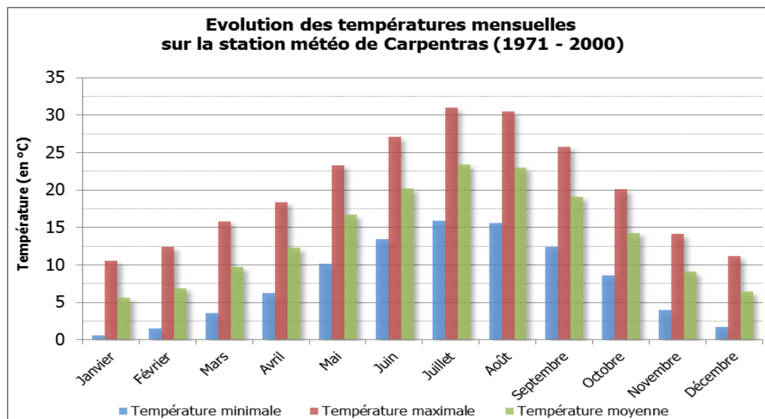
Figure 2 : Evolution des températures mensuelles (station de Carpentras)
