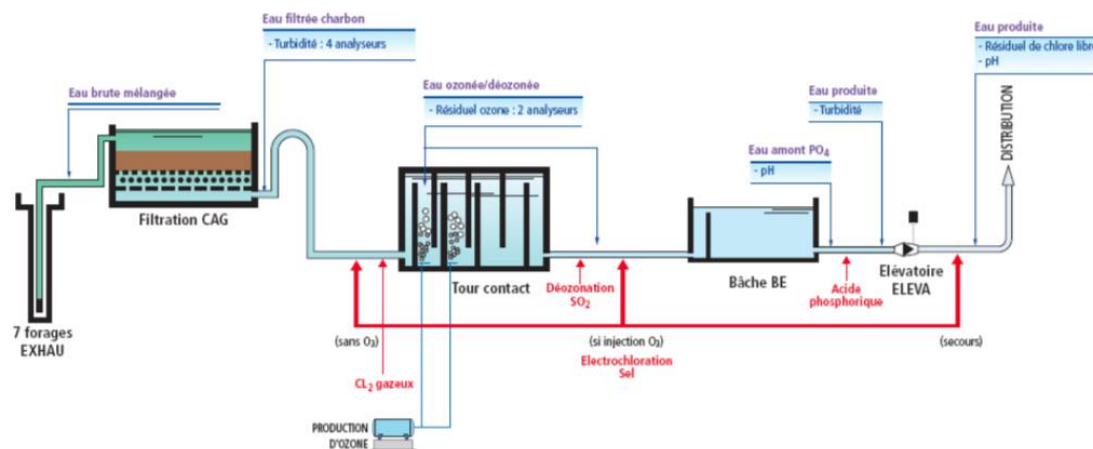
Schéma de fonctionnement de l'usine d'Arvigny (SEDIF)
