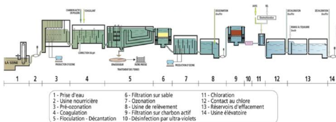
Schéma de fonctionnement de l'usine de Choisy-le-Roi (SEDIF)
