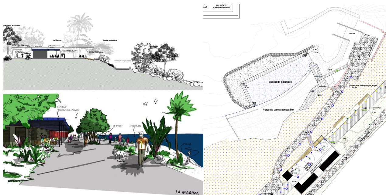
Plan d'avant-projet présentant le bassin de baignade, l'abri côtier et la marina. Coupe et illustration d'ambiance de la marina présentant ses jardins et son pôle de restauration – ces documents n'ont pas de valeur réglementaire
