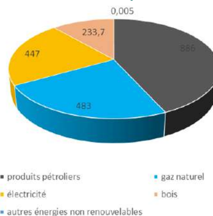
Mix énergétique du PETR en GWh/an tous secteurs confondus
